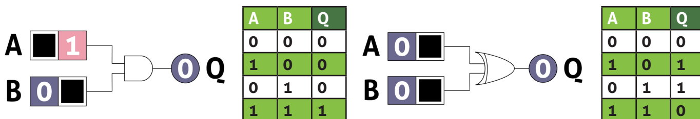
Estrebou, Mesía, & Sanz, 2017 (Redibujado por Lic. Edward Trinidad)
